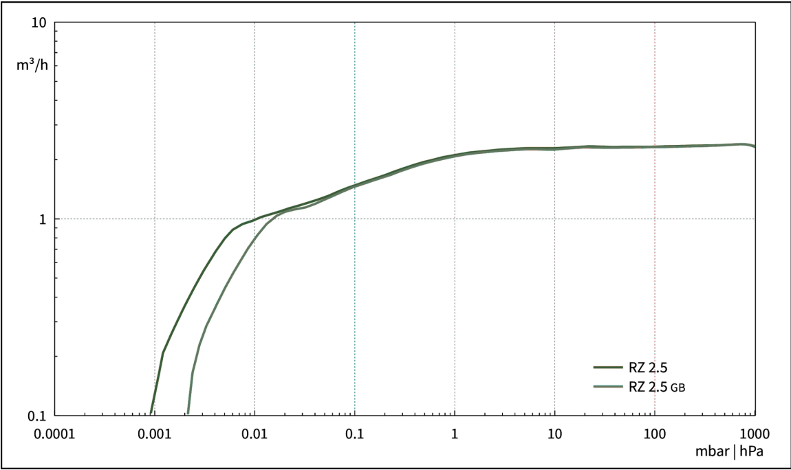
Curva de bombeo en 50 Hz (Volumen 10 l)
